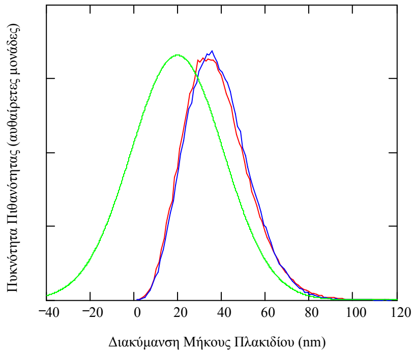
Σχήμα 2. Πυκνότητα πιθανότητας της διακύμανσης μήκους πλακιδίου, με v_{\text{eff}}=27 ενεργούς βαθμούς ελευθερίας (κόκκινη γραμμή), για v_{\text{eff}}=\infty (μπλε γραμμή), και για τον υπολογισμό της εξίσωσής 7 (πράσινη γραμμή).
